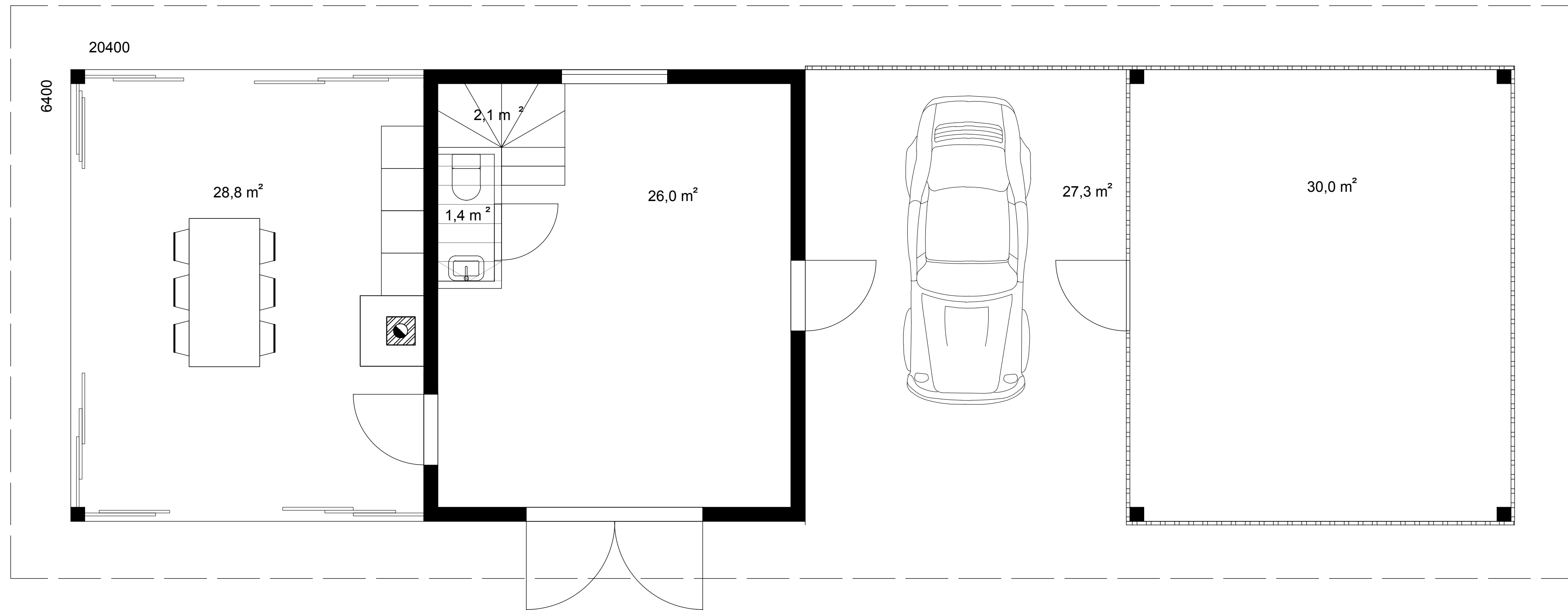
Põhikorrus/Ground floor
