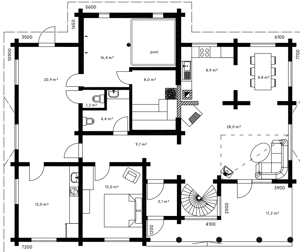
Põhikorrus / Ground floor
