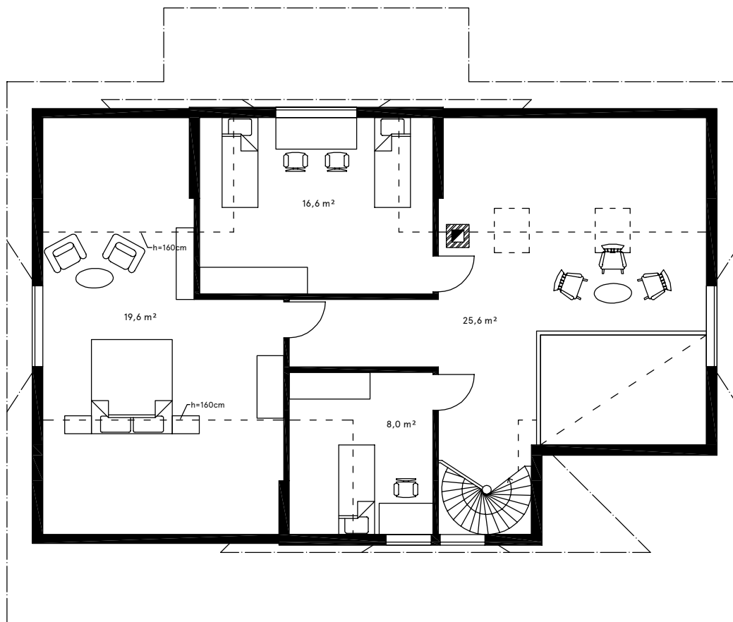
Katusekorrus / Upper floor
