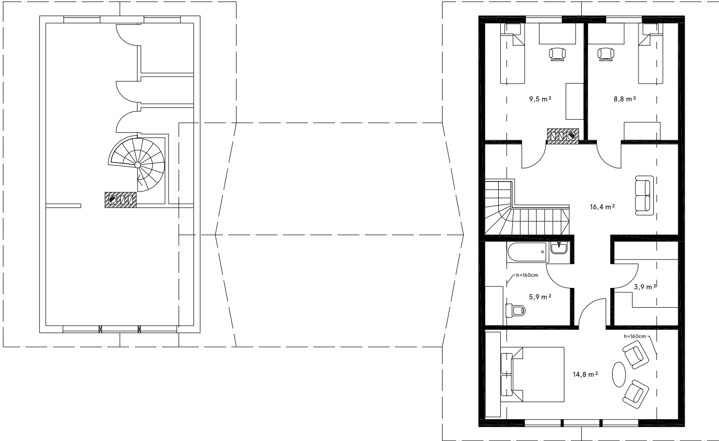
Katusekorras / Upper floor
