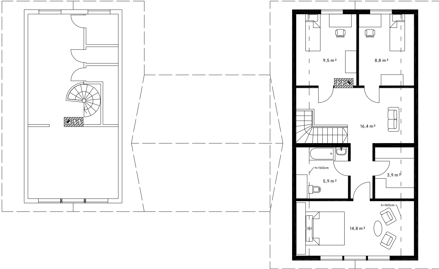
Katusekorros / Upper floor
