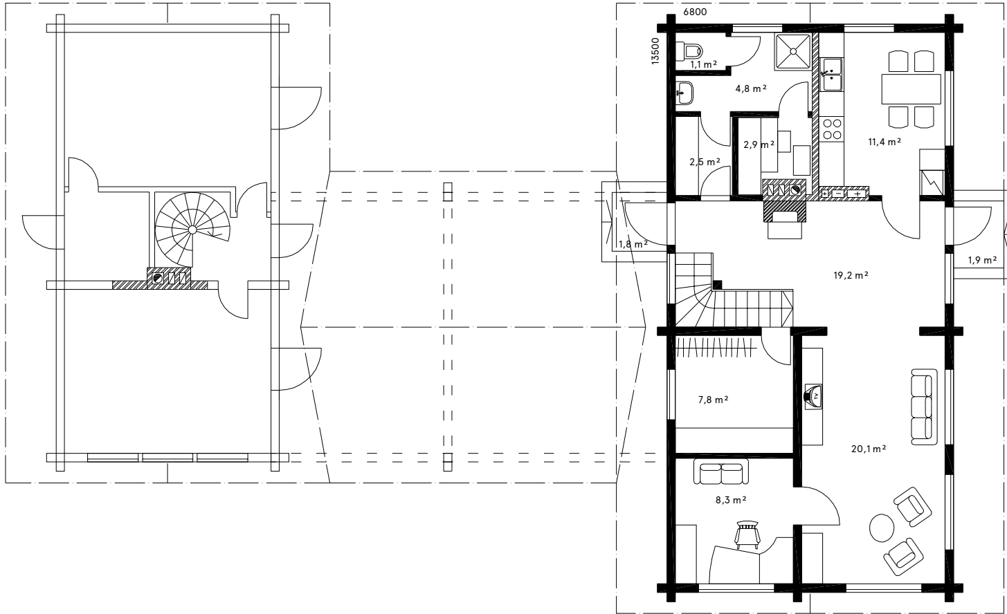
Põhikorrus / Ground floor
