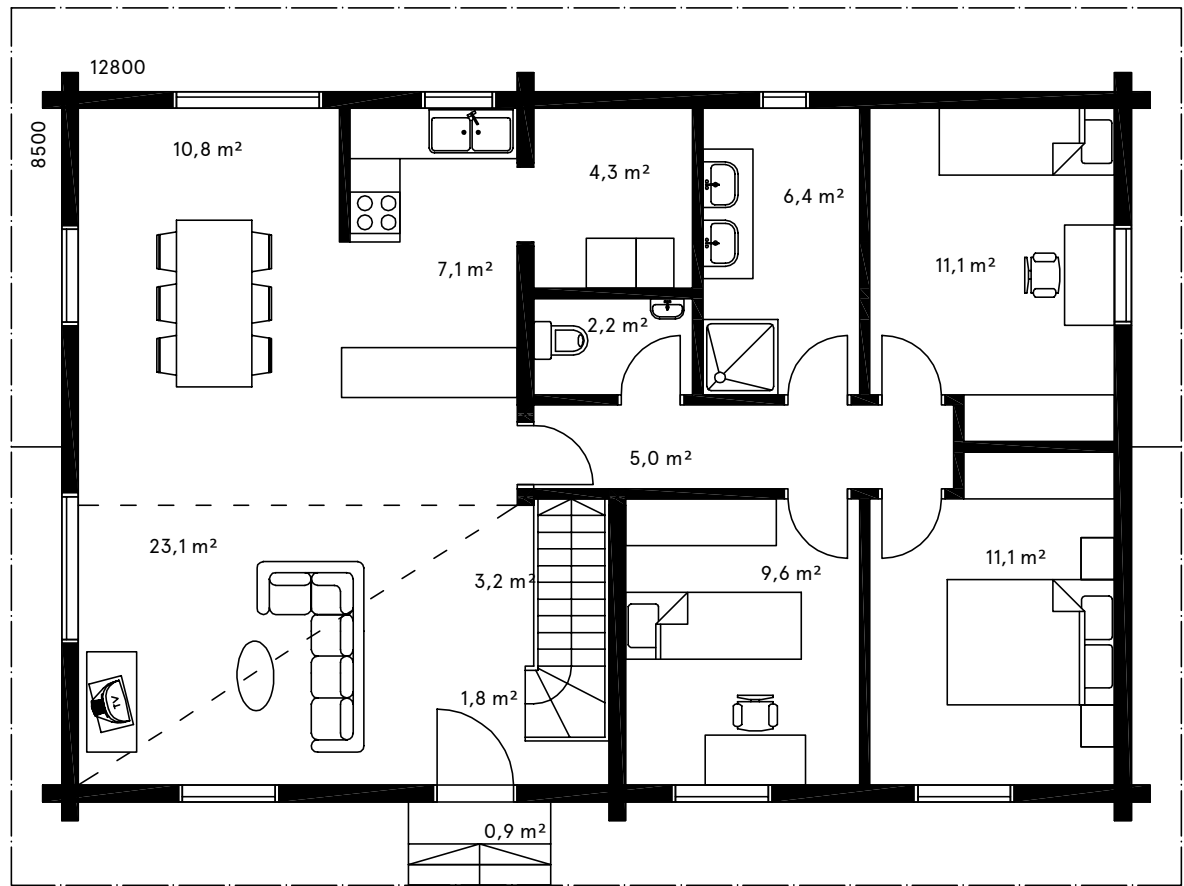
Põhikorrus / Ground floor
