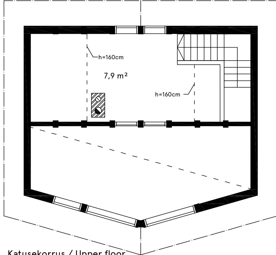
Katusekorrus / Upper floor
