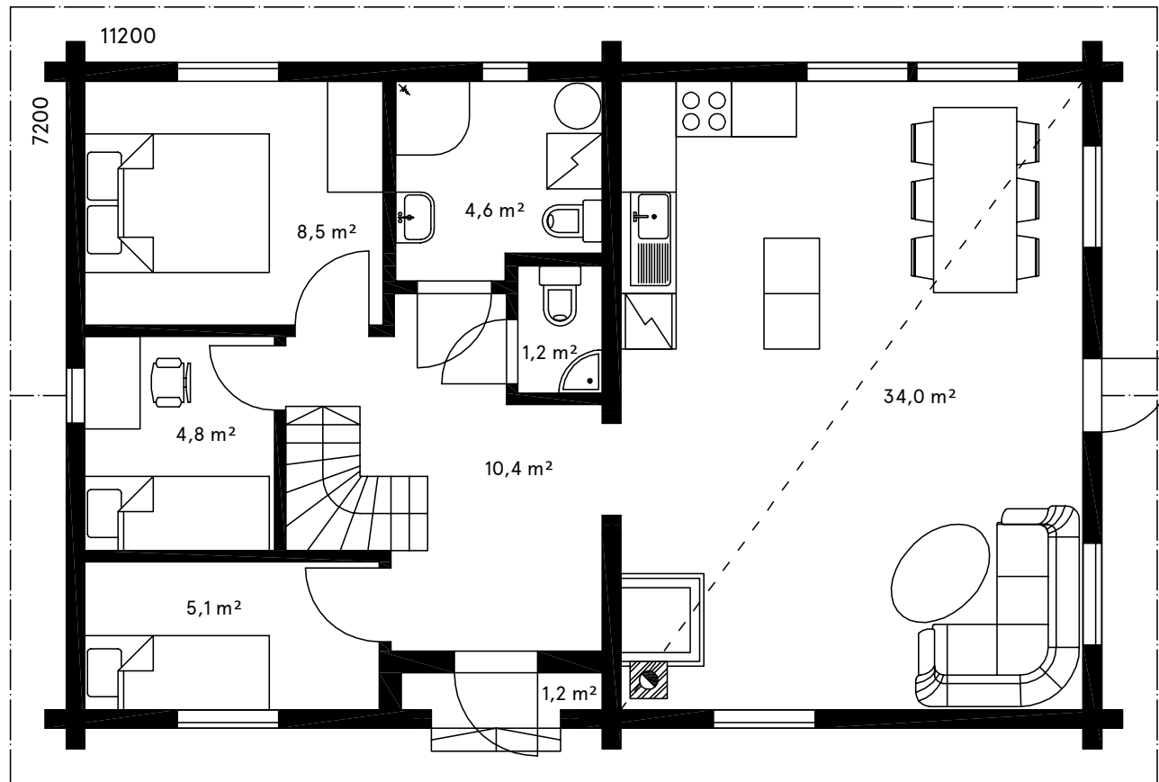
Põhikorrus / Ground floor
