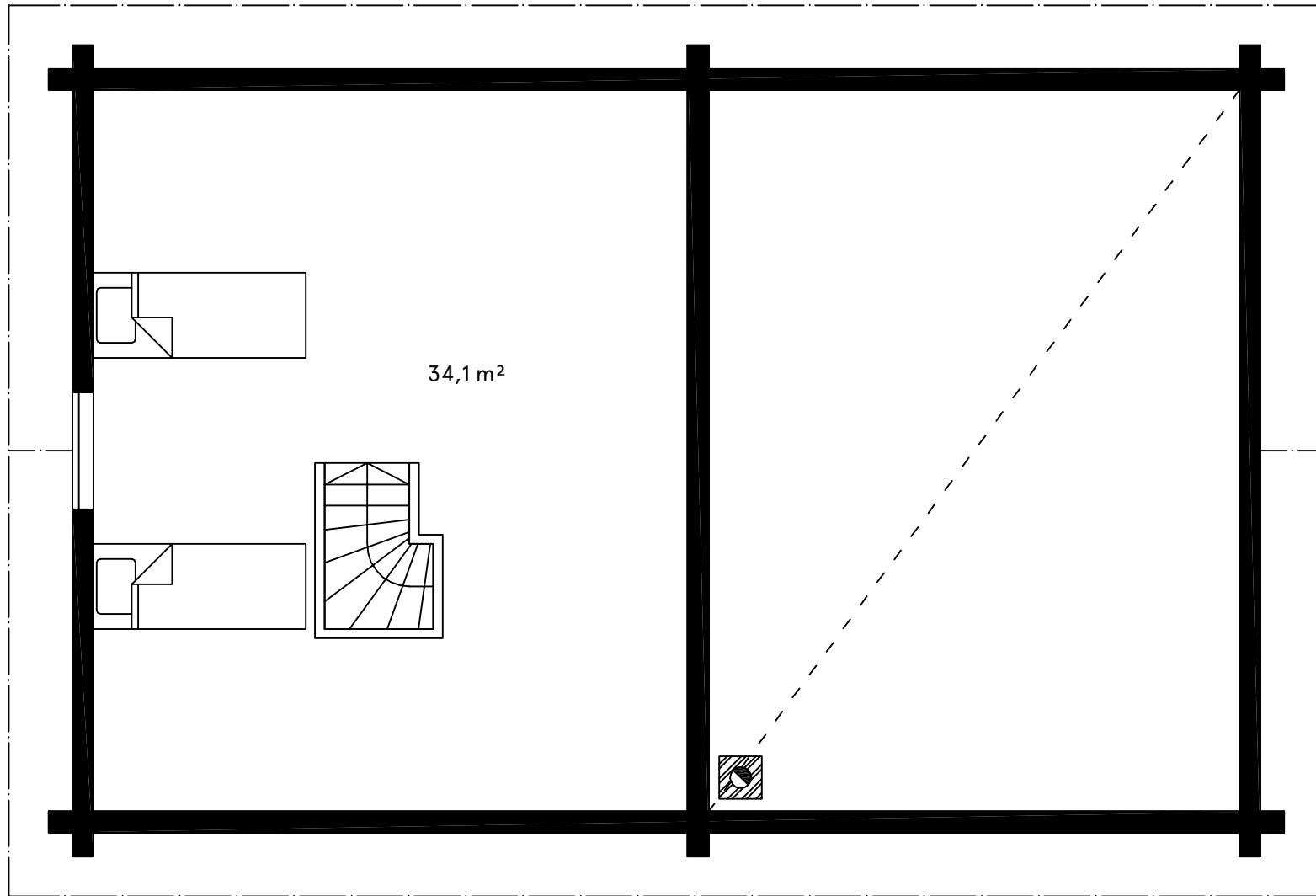
Katusekorrus / Upper floor
