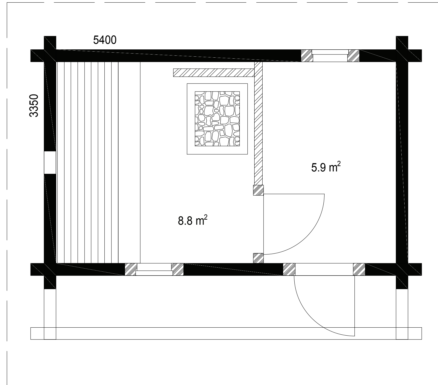
Põhikorrus/Ground floor
