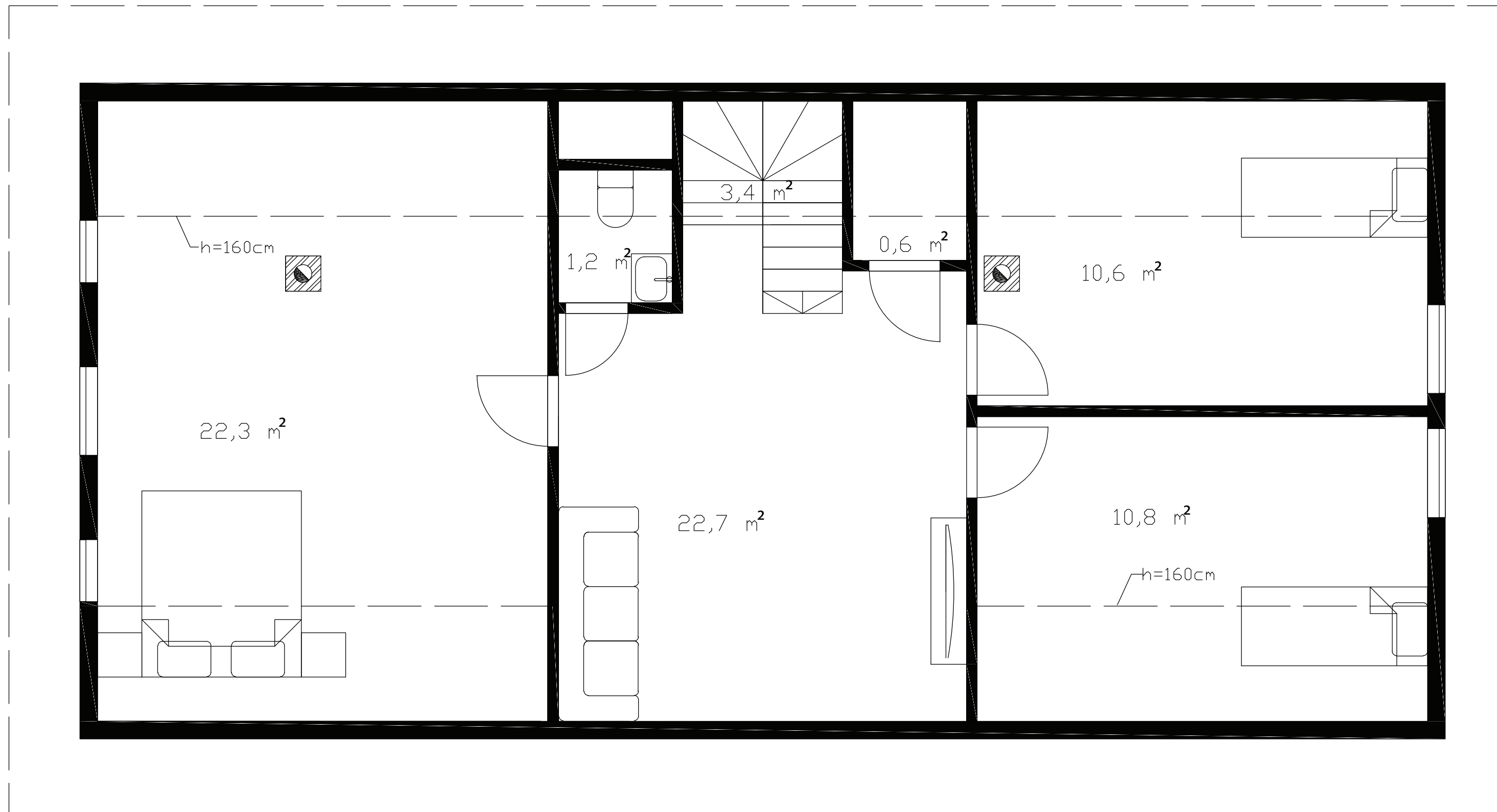
Katusekorrus/Upper floor
