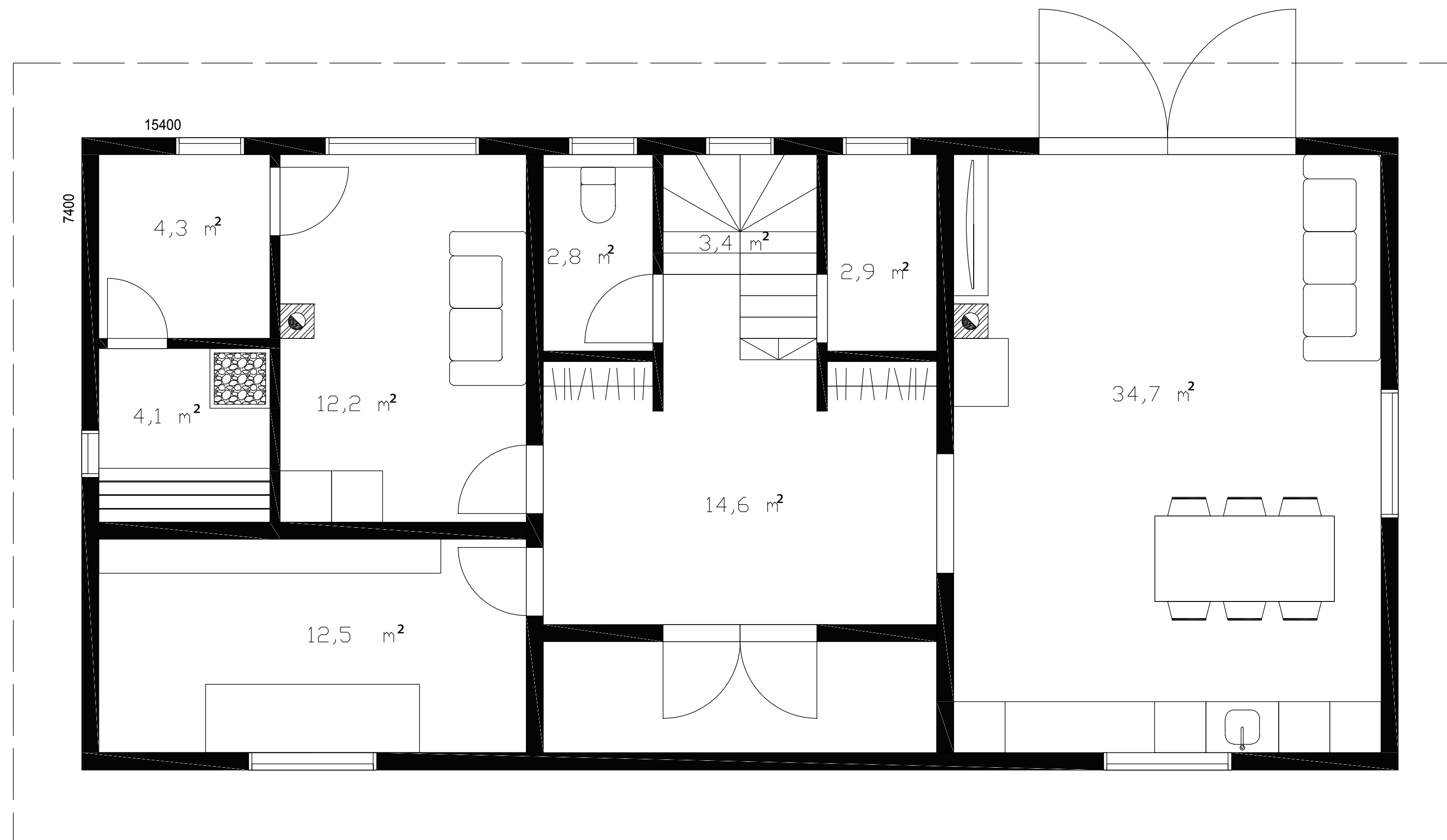
Põhikorrus/Ground floor
