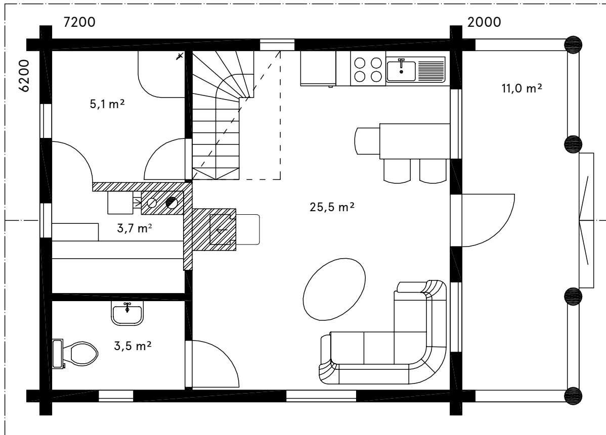
Põhikorrus / Ground floor
