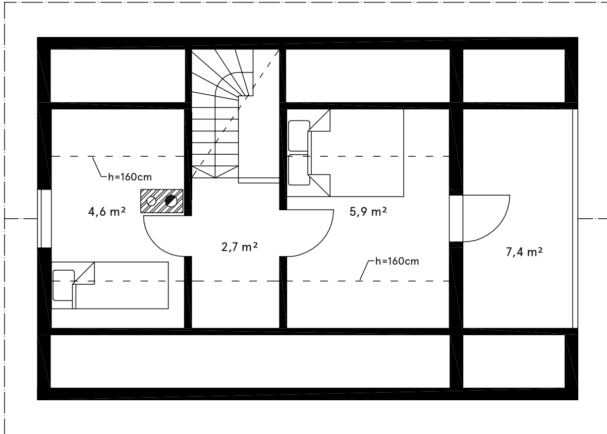
Katusekorrus / Upper floor
