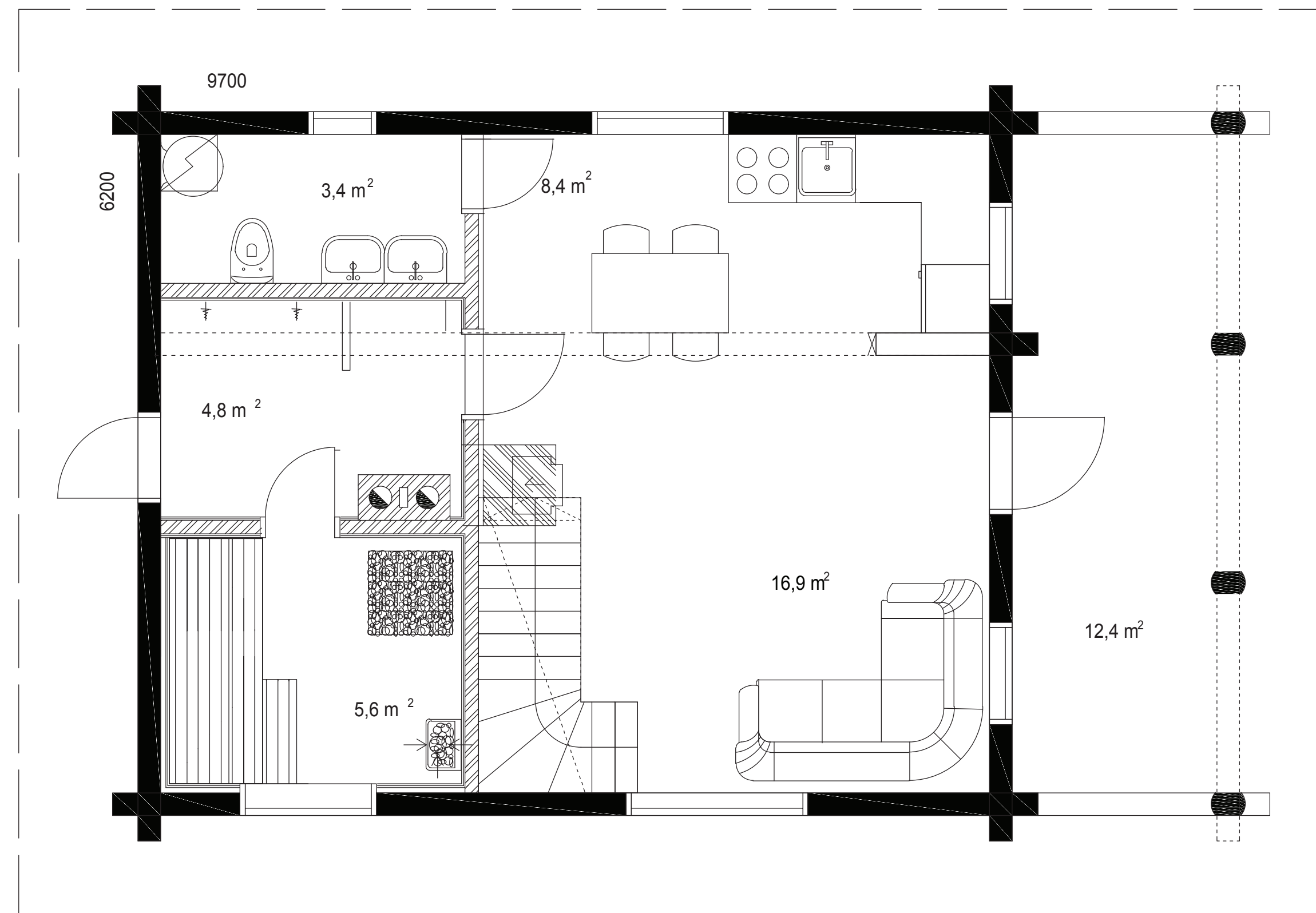
Põhikorrus/Ground floor
